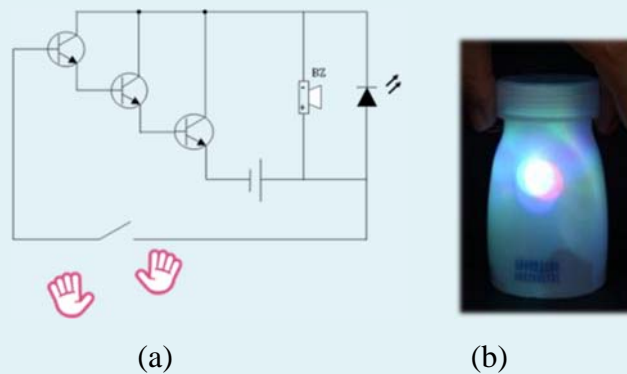
圖 2 本科普團隊研發之能量罐或稱嗶嗶罐 DIY 實驗的(a)電路示意圖和 (b)實體成品。
